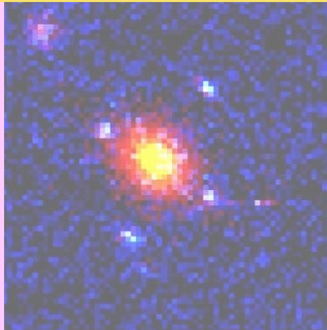
Immagine di una "lente gravitazionale", che visualizza immagini multiple di un oggetto centrale (cf. www.pd.astro.it/MOSTRA/NEW/A9002STR.HTM )
